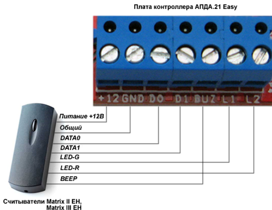
Рисунок 3 – Схема подключения считывателей
